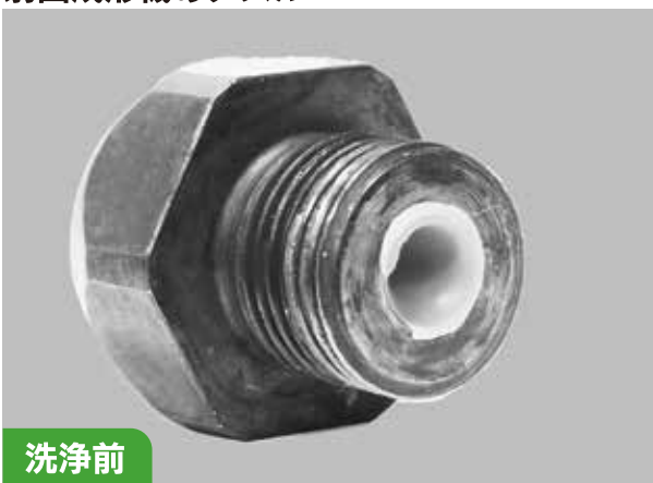
射出成形機のノズル
