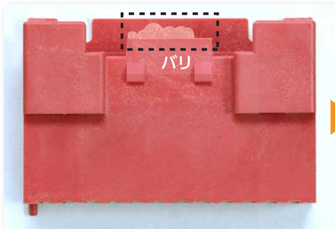
バリが発生した成形品
